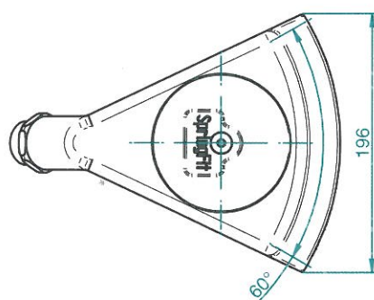
Fingerstrahldüse 25-4 Art.-Nr.: 4822150
