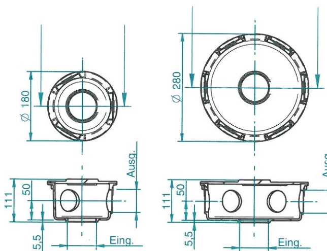
Wasserverteiler ø150mm Art.-Nr.: 4824050 Art.-Nr.: 4824150 Art.-Nr.: 4824250
