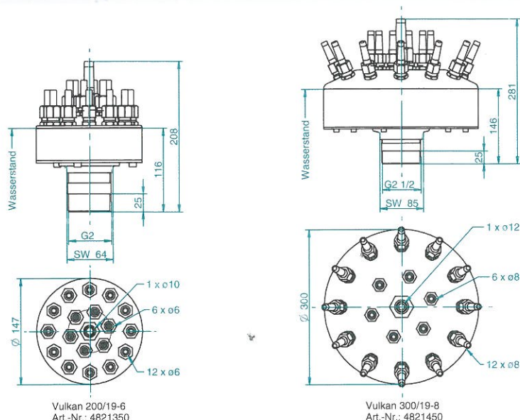
Vulkandüse 200/19 - 6 Volcano nozzle 200/19 - 6 4821350
