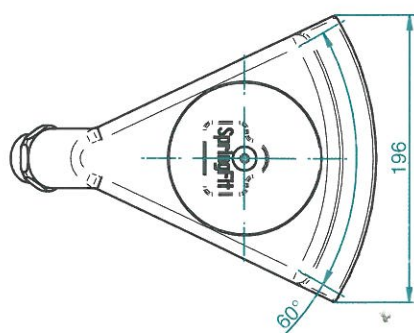
Fingerstrahldüse 13-4 Art.-Nr.: 4822050
