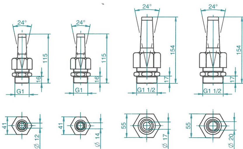
Komet 10-12 Art.-Nr.: 4823450
